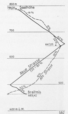
Abb. 2. Längenprofil 1 : 7000/7000
