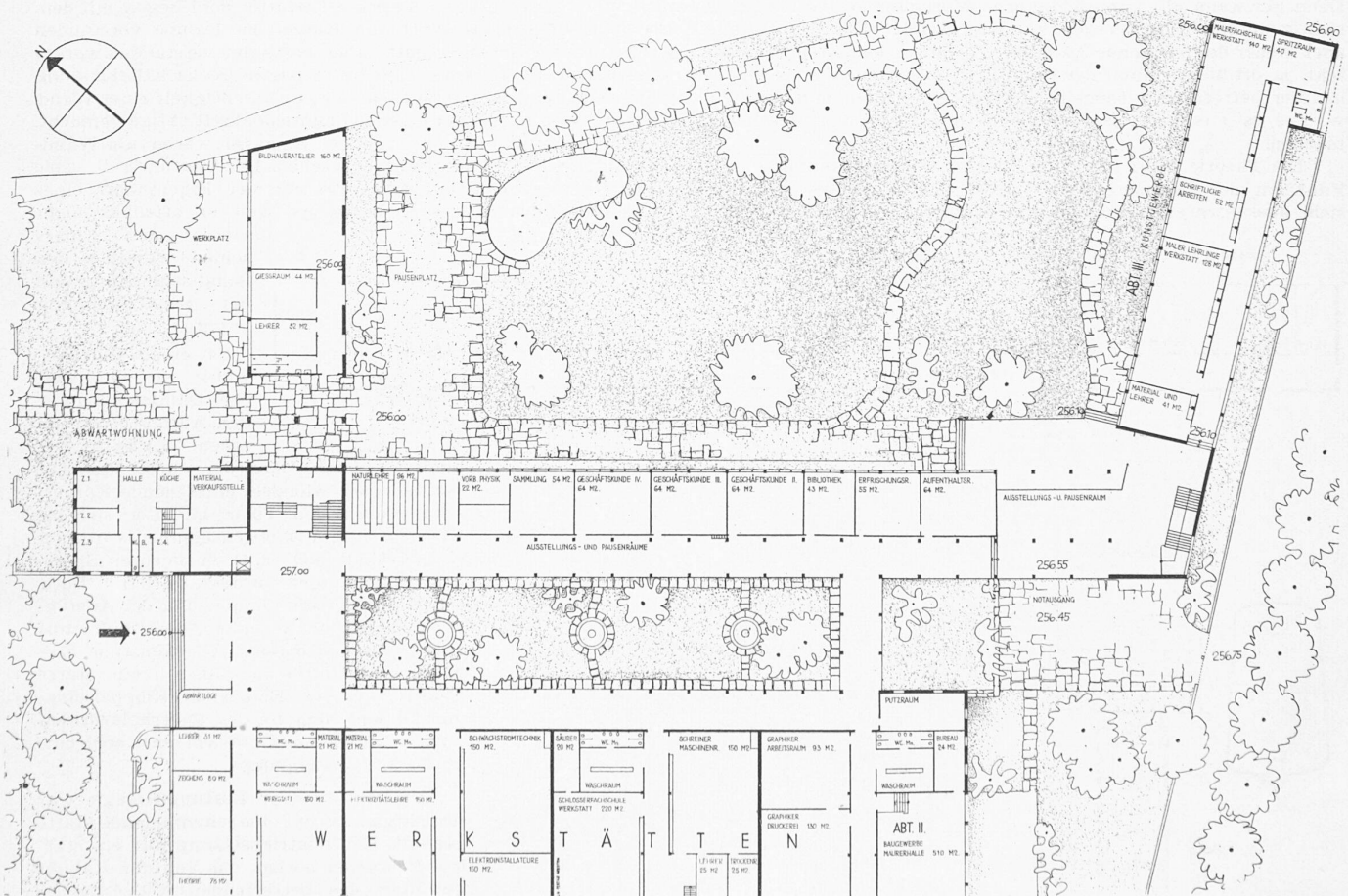
1. Rang (5500 Fr.), Entwurf Nr. 26. Verfasser BRAUNING, LEU, DÜRIG, Architekten, Basel. — Erdgeschoss 1 : 800, oben Isometrie
