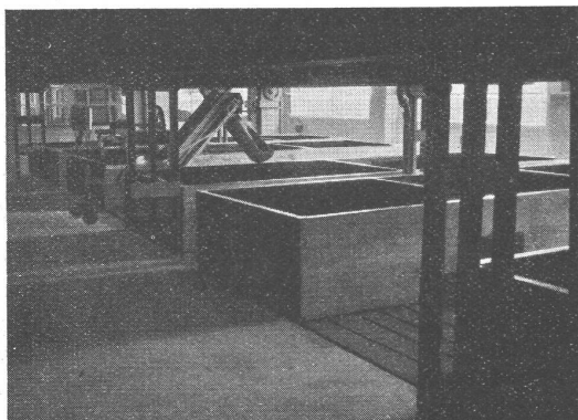
14 Sauerkrautbehälter der Firma Sturzenegger & Schiess AG. Zürich, mit „Gaschell 4“ ausgekleidet.
