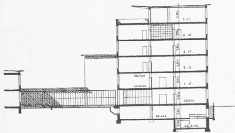
Schnitt Hochbau 1 : 800
