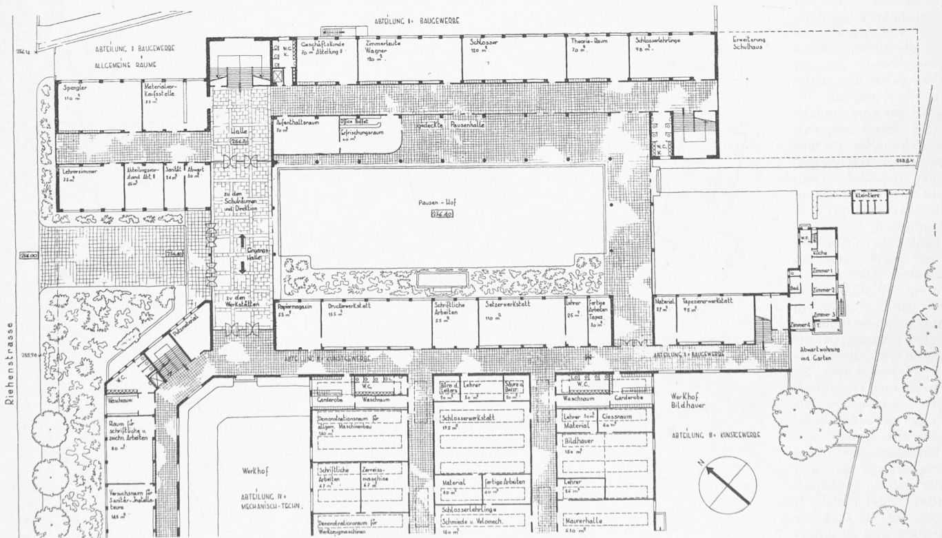
Unten Erdgeschoss, 1 : 800
