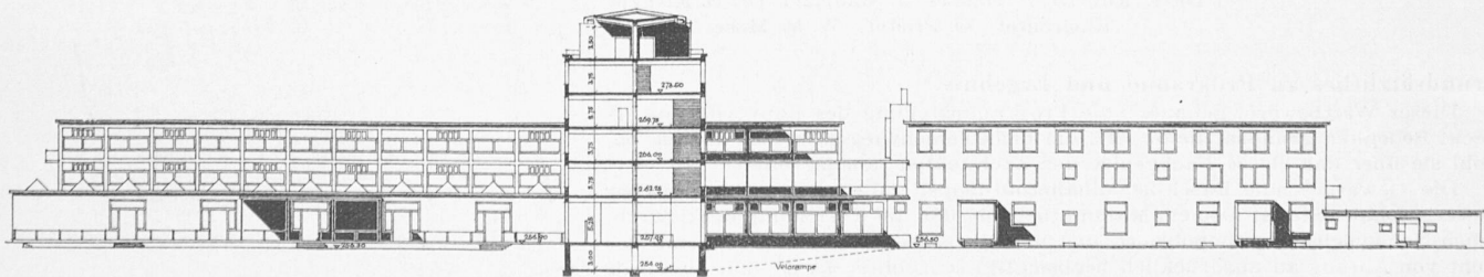
LÄNGSSCHNITT IN DER MITTELAGSE
