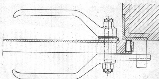
Abb. 3. Schlosseite mit Riegelverschluss, geschlossen Schnitte, Masstab 1:5
