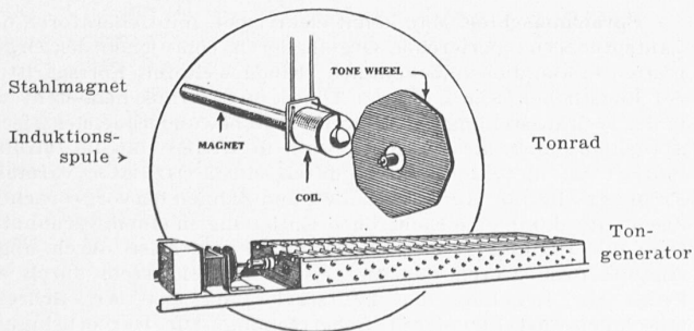
Abb. 14. Schema des Tongenerators der Hammond-Organ
