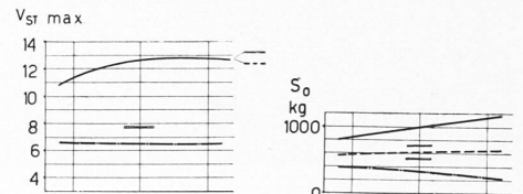
Abb. 1a. Höchst- und max. Steiggeschwindigkeit
