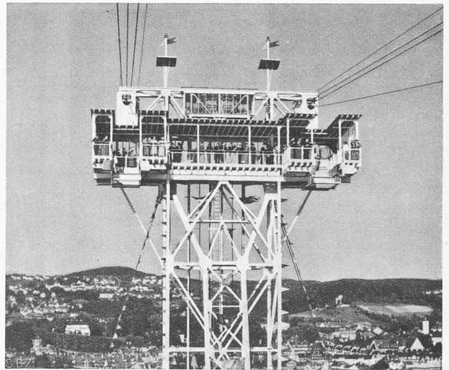
Abb. 49. Turmkopf rechtes Ufer, gegen den Zürichberg
