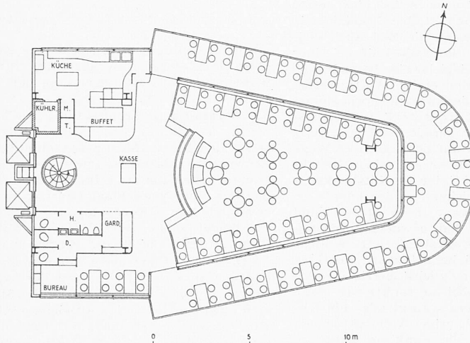
Abb. 46. Turmrestaurant. — Alle Grundrisse 1 : 250
