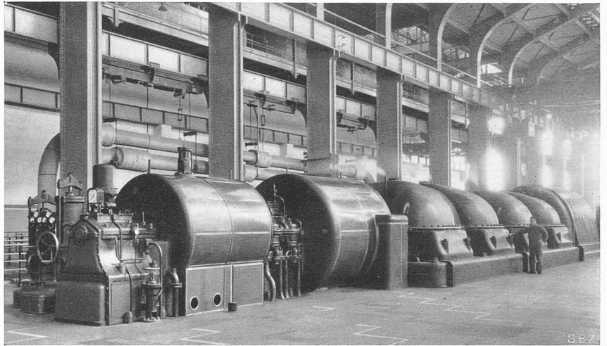
Abb. 1. Vierzylinder-Dampfturbine Oerlikon für 50000 kW, 55 at, 450° C, 300 U/min in der Zentrale St. Denis II, Paris. (Eingehend beschrieben in «SBZ», Bd. 110, S. 235*)
