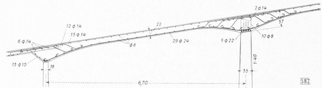
Abb. 6. Armierung, 1 : 120
