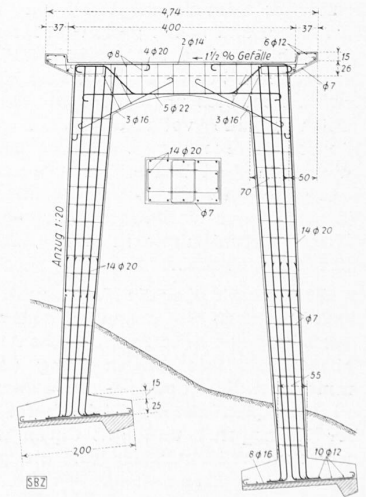
Abb. 7. Brückenjoch 1 : 120
