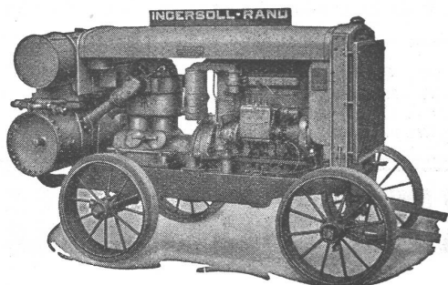
Rohölkompressor 20/26 PS.
