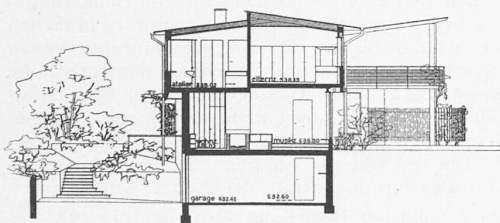
querschnitt
