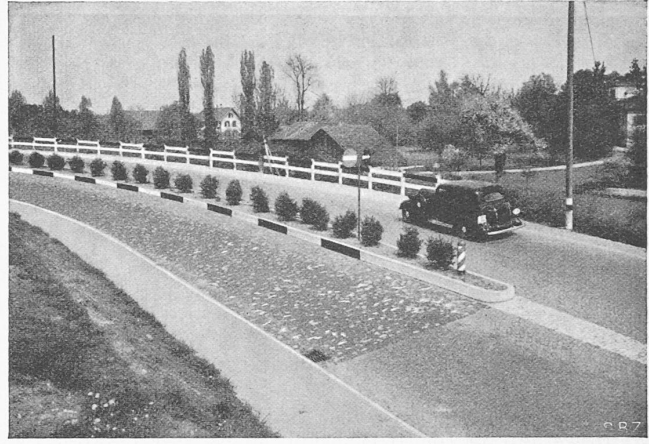
Abb. 2. 50 m-Kurve der st. gallischen Staatstrasse St. Gallen-Rorschach Gehweg 2,0 m, 2 Fahrbahnen je 5,0 m, Grünstreifen 2,0 m, Quergef. 7 ‰
