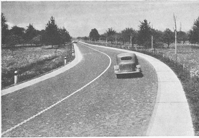
Abb. 1. 100 m-Kurve der st. gallischen Staatstrasse St. Gallen-Bauriet Fahrbahnbreite (dunkel) 9 m, helle Radfahrwege je 1,25 m, Quergef. 8 ‰
