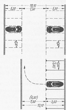
Abb. 4. Garagen, oben (zweibündig) auf Standplätzen, unten in Boxen
