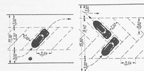
Abb. 2. Standplätze in Schrägaufstellung Abb. 3 (rechts) in Senkrechtaufstellung
