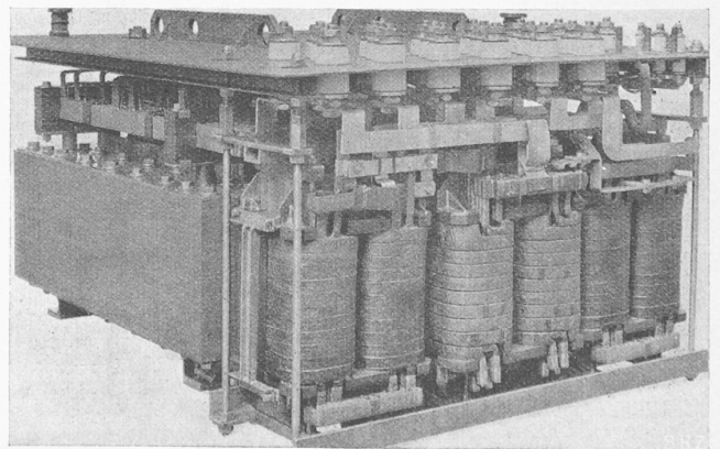
Abb. 4. Transformator mit Uberschaltspulen, ohne Oelkessel
