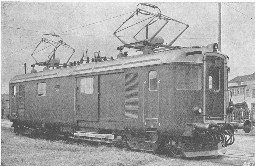
Abb. 3. Leichter elektr. Gepäcktriebwagen der SBB, gebaut von «SLM-Winterthur» und «Oerlikon» Gewicht 52 t, Stundenleistung 1340 PS (= 3880 kg am Radumfang), V_{\max} = 125 km/h
