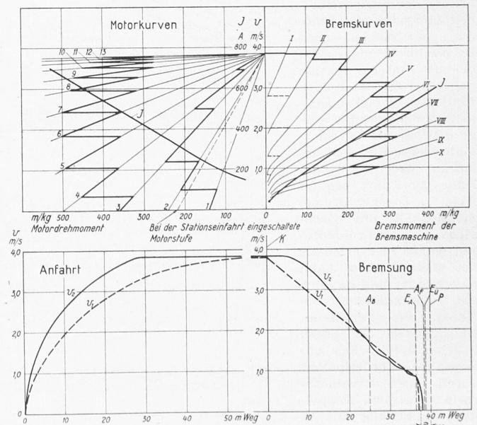
Abb. 20. Fahrdiagramm der II. Sektion bei automatischem Betrieb Legende: a mittl. Abstand zwischen Wagen- u. Stationspuffer 2,54 m, A B bewegl. Anschlaghebel, EA Abschaltung durch Endausschalter, A F fester Anschlaghebel, Eu Endumschalter, P Pufferbalken, K Kontakt am Wagenstandanzeiger, v 1 Fahrgeschwindigkeit bei Anfahrt und Bremsung mit max. Ueberlast bergwärts, v 2 desgl. talwärts
