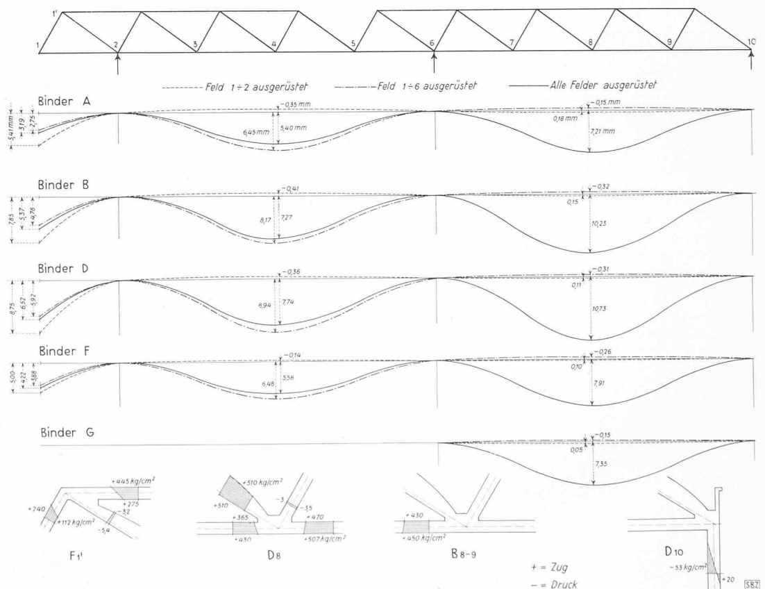
Abb. 15. Biegelinien und Spannungen im Schalenshed-Tragwerk von 2 \times 27 m Stützweite ermittelt bei Absenkung des Gerüsts am 6. Januar 1938 (Lage und Bezeichnung der Binder vergl. Abb. 4)
