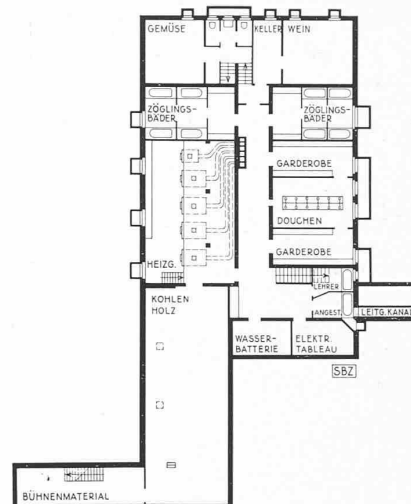
Abb. 11. Kellergrundriss 1 : 500
