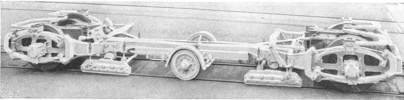
Abb. 6. Dreilachsiges Lenkuntergestell der Schweiz. Lok.- u. Maschinenfabrik Winterthur
