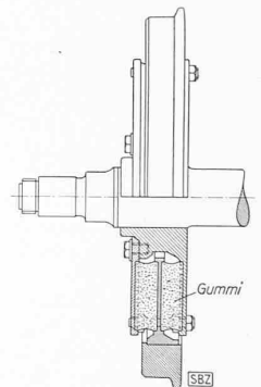
Abb. 8. Gummifederrad SAB
