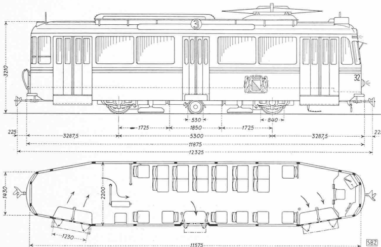
Abb. 5. Dreilachsiger Motorwagen. Tara 15,4 t, 180 kg/Platz. — 1:120
