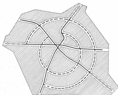
Abb. 1. Aufbau eines grossstädtischen Verkehrsnetzes (Schema)
