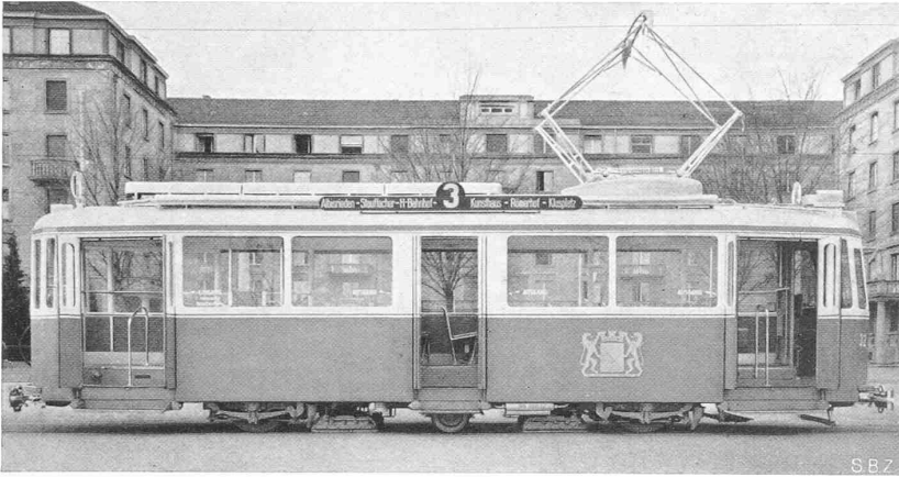
Abb. 7. Dreilachser der St. St. Zürich in Leichtstahlschalenbauart SWS Schlieren
