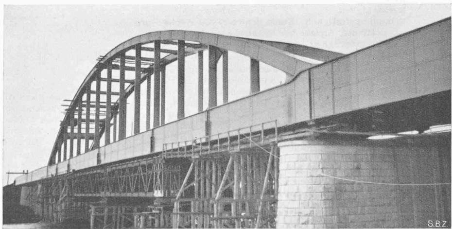
Abb. 1. Ansicht von der stromabwärtigen Seite der neuen zweigleisigen Eisenbahnbrücke der Jugoslawischen Staatsbahn über die Save bei Zagreb, erbaut 1937/39. — Biegunsfester, versteifter Stabbogen von 135,54 m Stützweite Linksufrig eine Seitenöffnung von 57,50 m, rechtsufrig zwei Öffnungen von 57,96 und 55,0 m
