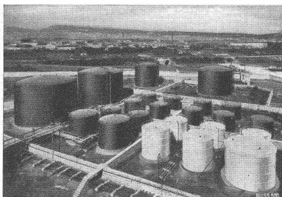
Erdöl- und Benzintankanlage von 30 000 m³ Gesamtinhalt, nach Neapel geliefert
