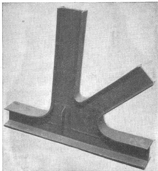
Autogen geschweisster Knotenpunkt.
