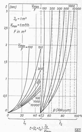
Abb. 10. Evakuierung eines Behälters mit gleichzeitigem Luftzutritt. Behältervolumen J_0 = 1 \text{ m}^3 Ansaugvolumen V_{\max} in m³/h Querschnitt des Luftzutrittes in m² Max. Vakuum der Pumpe p_2 = 0,02 \text{ ata}
