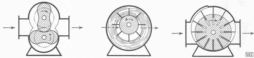
Kreiskolbengebläse
