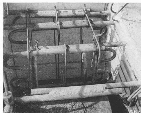
Abb. 44. Verschweisste und ergänzte Bewehrung in der Scheitelfuge, nach Herausnahme der Pressen
