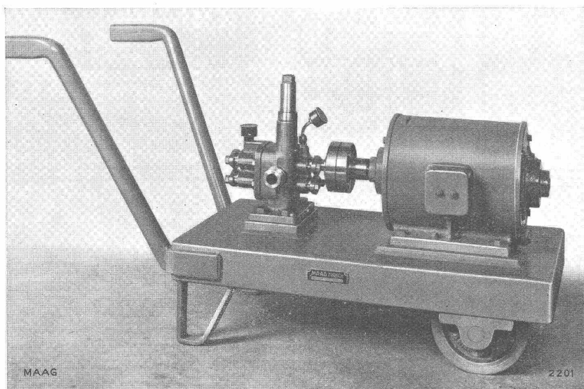
Fahrbare Maag-Zahnradpumpengruppe Type MP-35A zur Förderung von Fruchtsaft bei 12 Atm. Druck.
