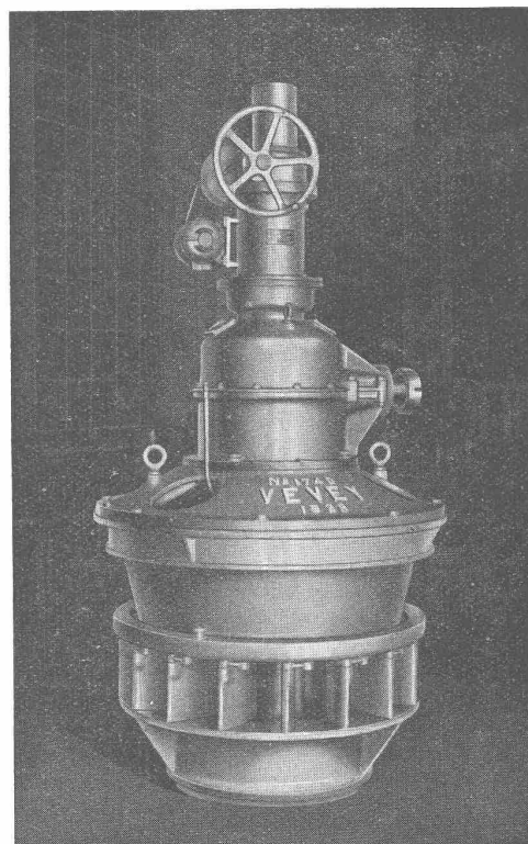
Kaplanturbine mit elektrisch gesteuerter Laufregulierung
