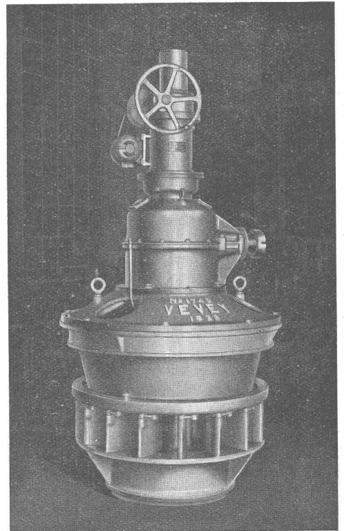
Kaplanturbine mit elektrisch gesteuerter Laufregulierung
