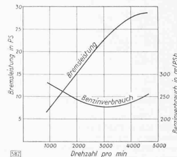
Abb. 5. Bremsleistung und Benzinverbrauch in gr/PSH in Funktion der Drehzahl
