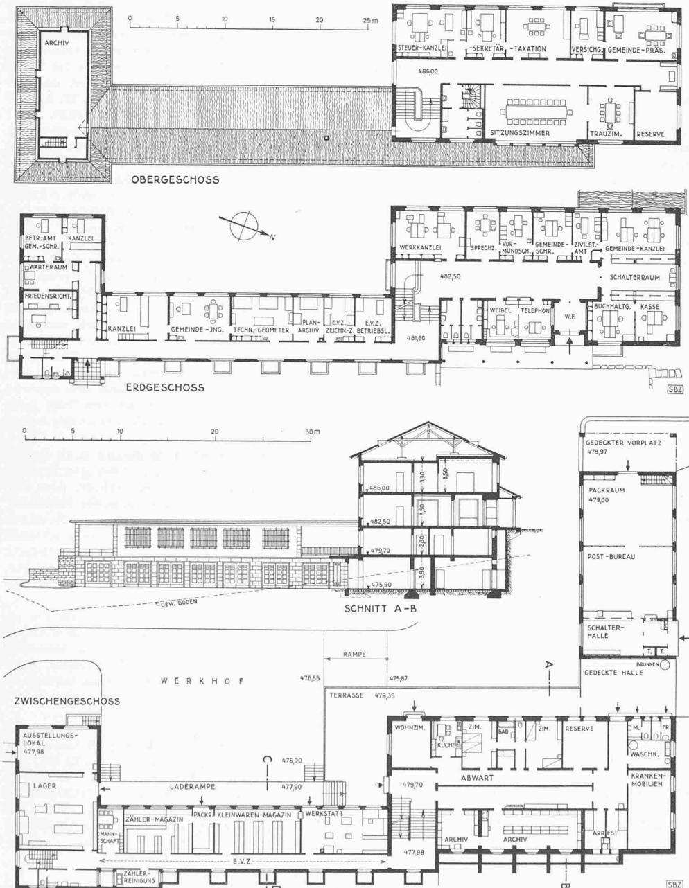
Abb. 6. Grundrisse und Schnitt A-B, Masstab 1 : 500
