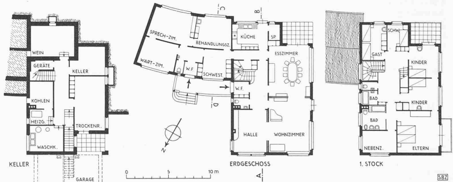
Abb. 2. Schnitte und Grundrisse. — Masstab 1 : 400
