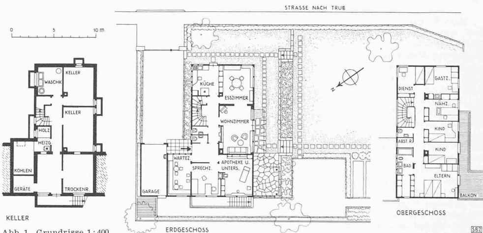
Abb. 1. Grundrisse 1:400
