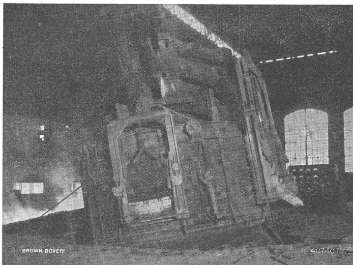
25-Tonnen-Stahlschmelzofen in Kippstellung
