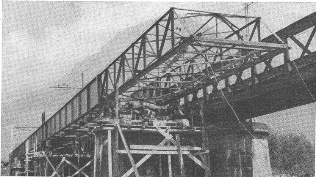
SBB eingleisige Bahnbrücke über die Moesa, Tessin
