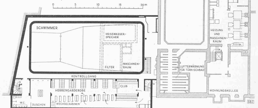
Abb. 1 (unten). Zweites Untergeschoss
