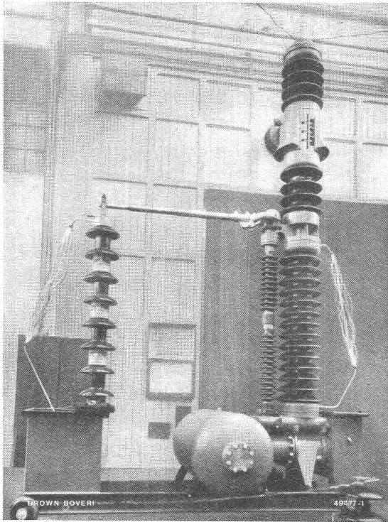
150 kV Druckluftschneiderschalter bei der Prüfung mit Stossspannung
