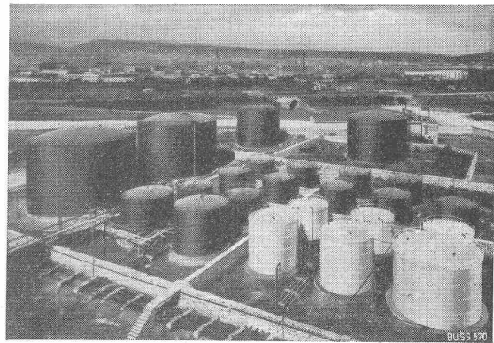
Erdöl- und Benzintankanlage von 30000 m³ Gesamtkapazität, nach Neapel geliefert
