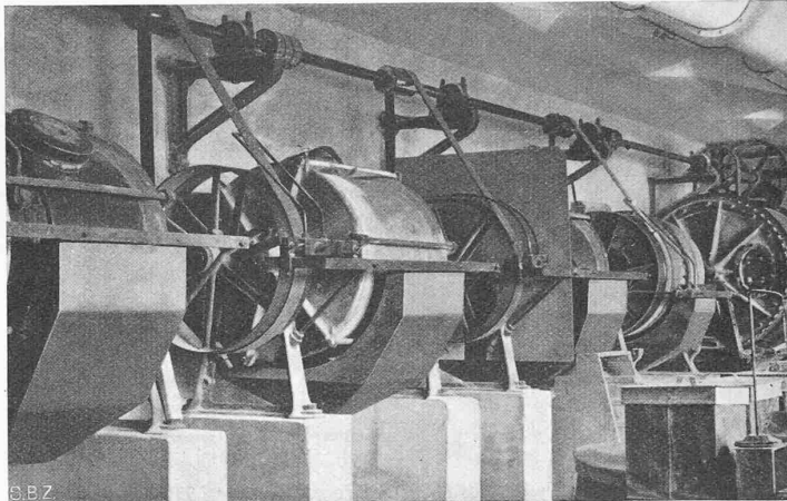
Abb. 2. Malen von körnigem Email in Kugelmühlen
