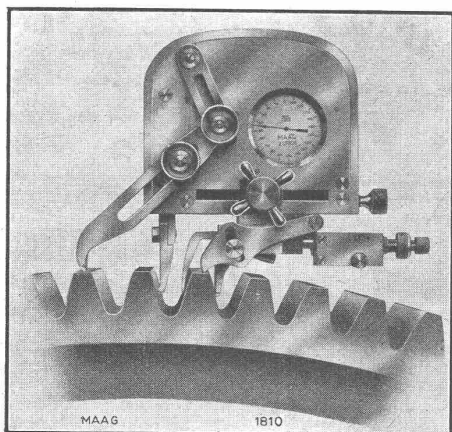
MAAG-Zahnteilungsmessgerät Type TMA, besonders für Kreisteilung.
