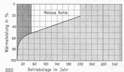
Abb. 1. Belastungs-Diagramm Jahresbetrieb Anteil der Raumheizung aus elektr. Energie (weisse Kohle) Anteil der Raumheizung aus Brennstoff (schwarze Kohle)
