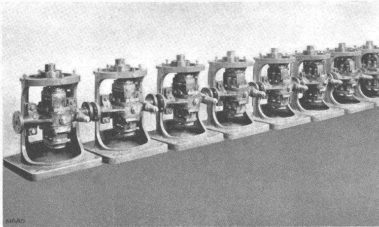
Gruppe vertikal gebauter Zahnradpumpen mit separaten Aussenlagern zur Förderung von Heisswasser für Schiffsbetrieb. Fördermenge: 67 l/m bei 6 Atm. Druck.
