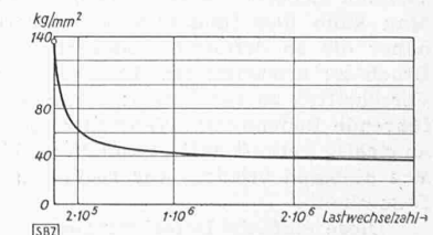
Abb. 3. Wöhlerlinie
