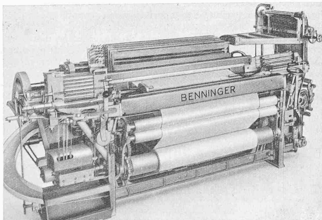
Abb. 28. Automatischer Seidenwebstuhl, Schützenwechsler
