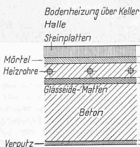
Abb. 17 und 18. Mustergültige Deckenquerschnitte eines zürcher. Bureaugebäudes. — 1 : 12
