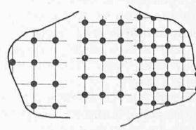
Abb. 13. Einige Typen gestörter Gitterordnung: links zwischen verschiedenen Kristallen schwankende Gitterkonstante, Mitte in ein und demselben Kristall schwankende Gitterkonstante, rechts Gitterstörung im Zusammenhang mit plastischer Verformung
