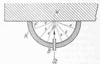
Abb. 4. Versuchsanordnung zur Aufnahme des «halben» Interferenzmusters. W das beliebig grosse Werkstück, F der Film, B die Blende zum Ausblenden des Strahlenbündels St, P der Aufnahmeort, 4 bis 6 die entstehenden Interferenzlinien, K die Kassette zum Schutz des Films gegen direkte Bestrahlung
