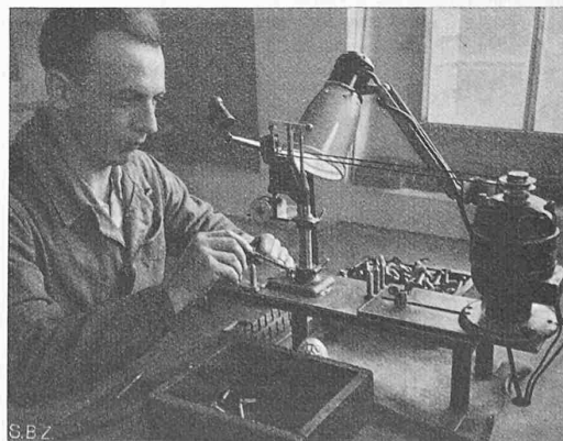
Bohren feiner Einspritzdüsenlöcher
