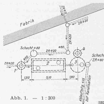
Abb. 1. — 1:300 1 Schlammfänger, 2 Belüftungsbecken, 3 Oelabscheider, 4 Oelsammler
