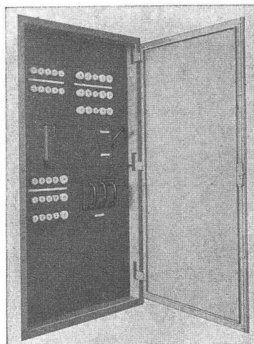
Schaltschrank putzbündige Montage
