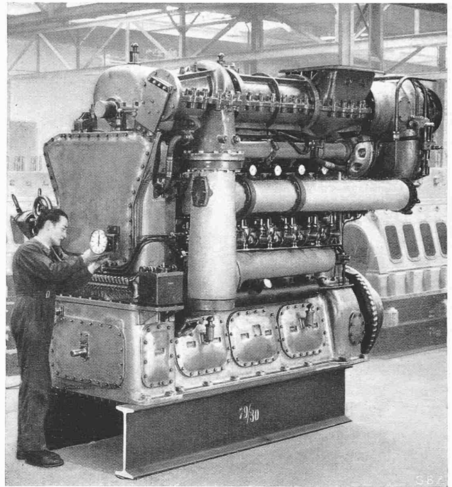
Abb. 18. Auf 2 ata aufgeladener Zweitakt-Zweiwellen-Gegenkolben-Sulzer-Dieselmotor von 1560 PS. Stundenleistung bei 850 U/min
