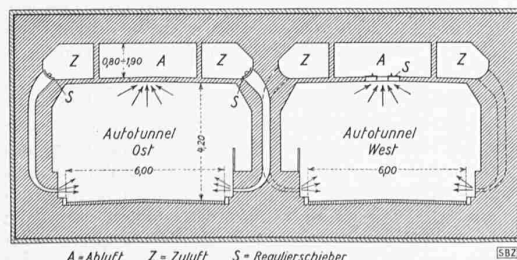
Abb. 11. Querschnitt Rampentunnel Abb. 12 (rechts). id. Flusstunnel
