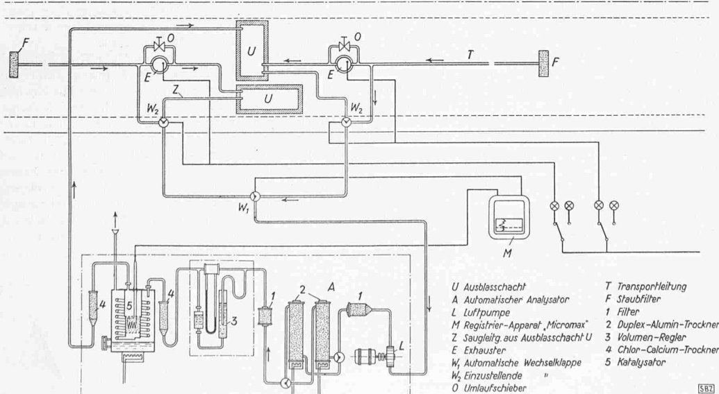
Abb. 14. Schema der CO-Messeinrichtung
