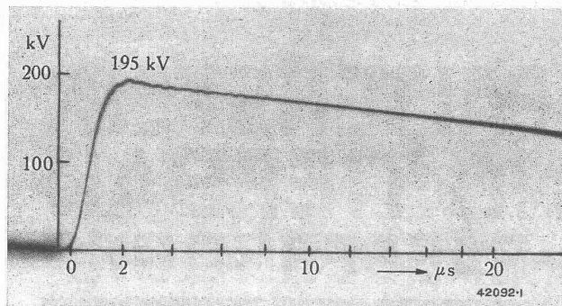
Verlauf des Spannungsschosses ohne Überspannungsableiter
