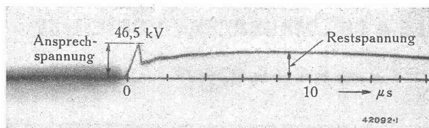
Verlauf des Spannungsschosses mit Überspannungsableiter
