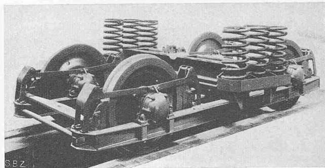
Abb. 1. Laufgestell mit Losrädern Bauart SLM Winterthur
